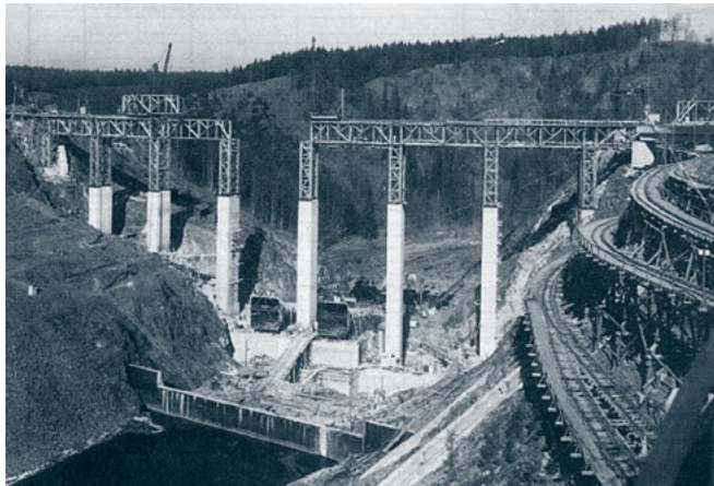
Bau der Bleilochtalsperre, um 1930
